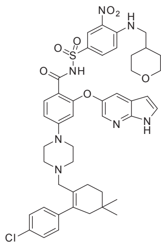
S804801, DMSO-d6
