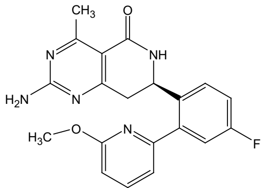
HSP-990 400MHz ^1\text{H} NMR DMSO- d_6
